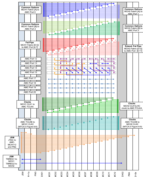
CMS Backplane Topologie
